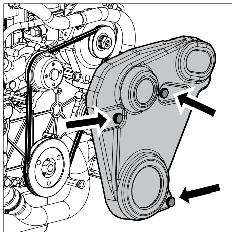
49 Keilriemenabdeckung entfernen
