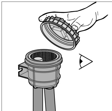
9 Kontrolle des Kühlwasserfilter
