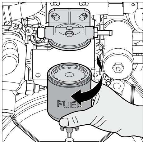
27 Kraftstofffilter abmontieren
