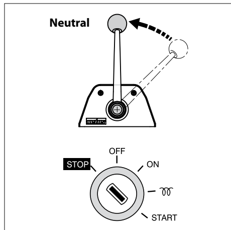
16 Stoppen
