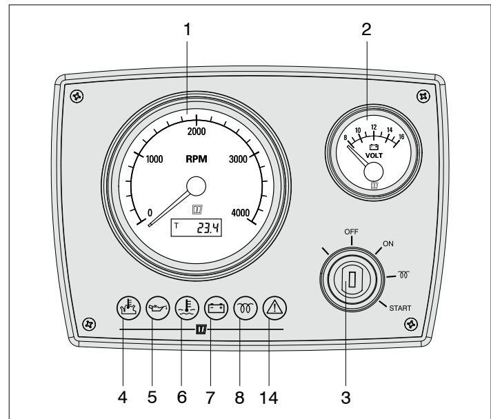
Steuerpult, Modell MPA22
