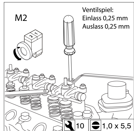
42 Einstellen des Ventilspiels
