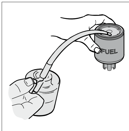
28 Kraftstofffilter montieren
