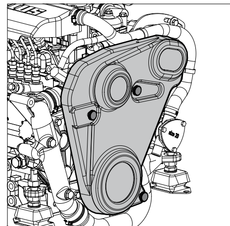
53 Keilriemenabdeckung anbringen
