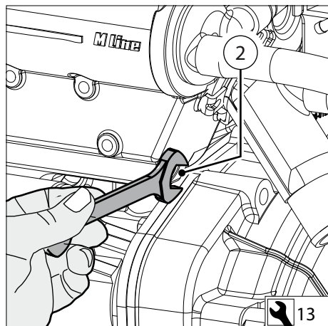
71 Entfernen der Ablaßschraube
