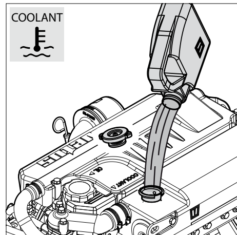
8 Nachfüllen Kühlsystem
