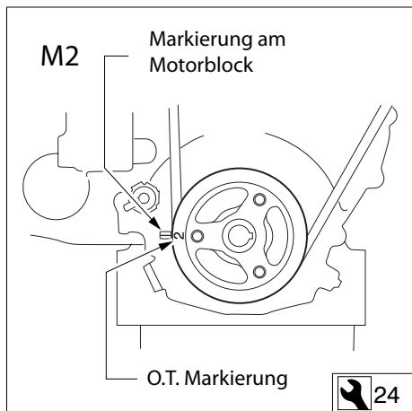
41 Bestimmung des O.T.
