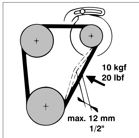
51 Kontrolle Spannung
