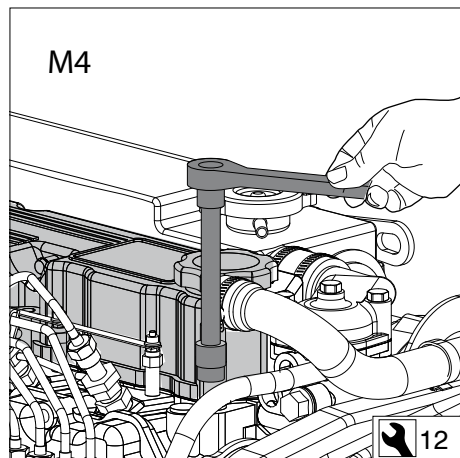
46 Ventildeckel entfernen
