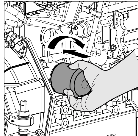
19 Ölfilter montieren
