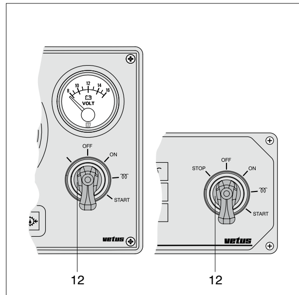
Steuerpult, Modelle MP10, MP22, MP34 nur für SOLAS-Motoren
