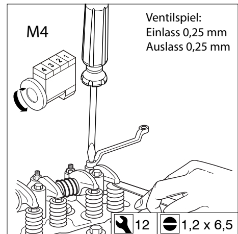
48 Ventilspiel einstellen
