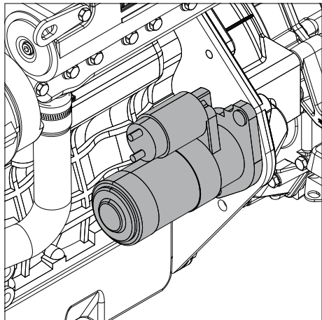
67 Anlasser kontrollieren
