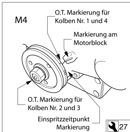
47 Bestimmung des O.T.
