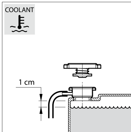
7 Kühlflüssigkeitsstand
