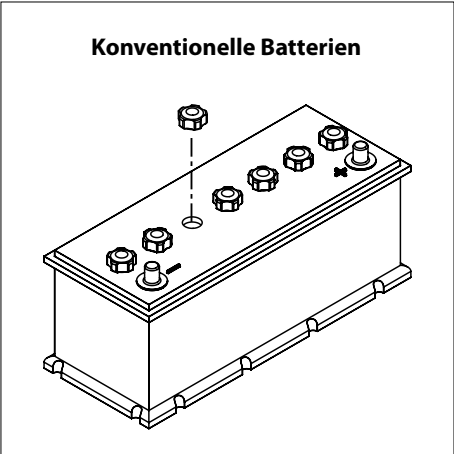
24 Kontrolle Pegel Batterieflüssigkeit
